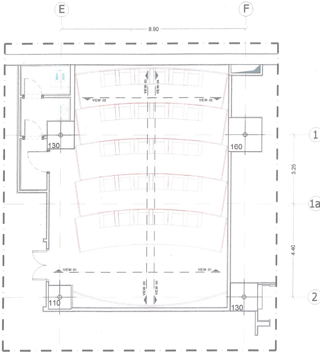
پلان بزرگنمایی سینما 13.15-
