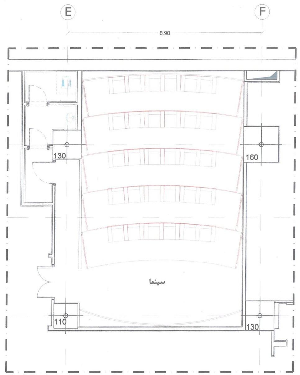
پلان مبلمان سینما 13.15-
