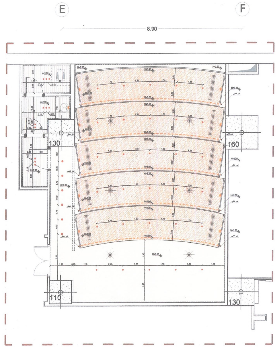
پلان سقف كاذب و روشنائى سينما 13.15-
