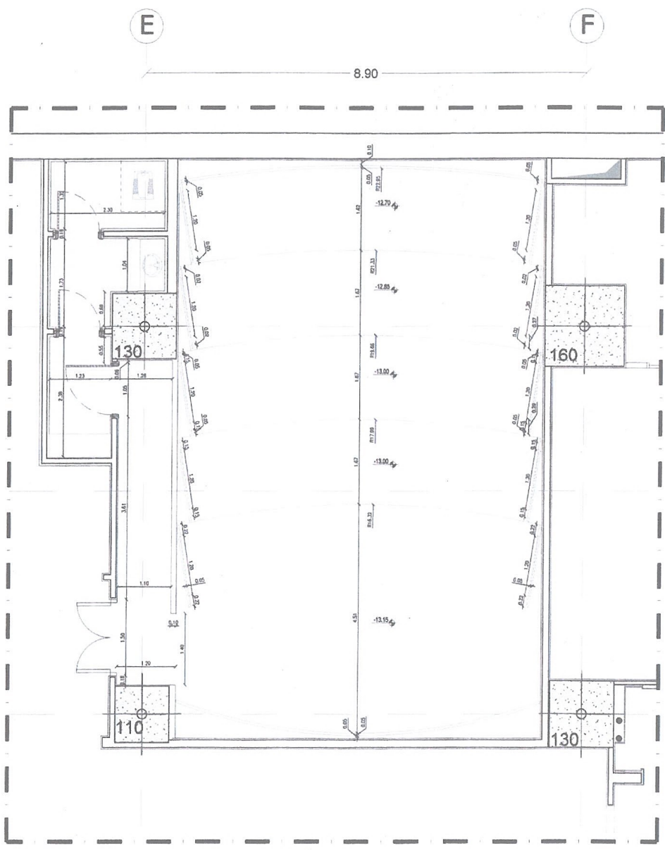
پلان اندازه گذاری سینما 13.15-
